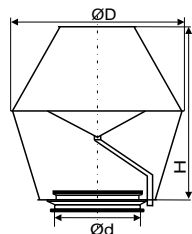
Deflektoriai HF (tvirtinami flanšu)
