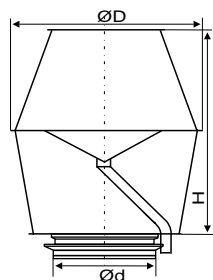
Deflektoriai HN (maunami ortak)
