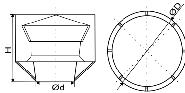
Deflektoriai T (nat raliai ventilacijai)
