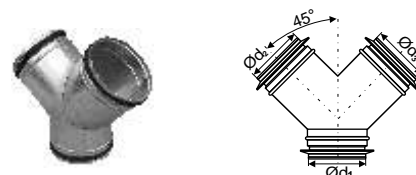
Kelnis YVU (su sandarinimo gumelėmis)
