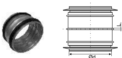
Movos NPU (su sandarinimo gumelėmis)
