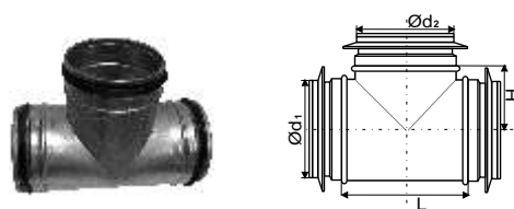
Trišakiai TCPU (su sandarinimo gumelėmis)
